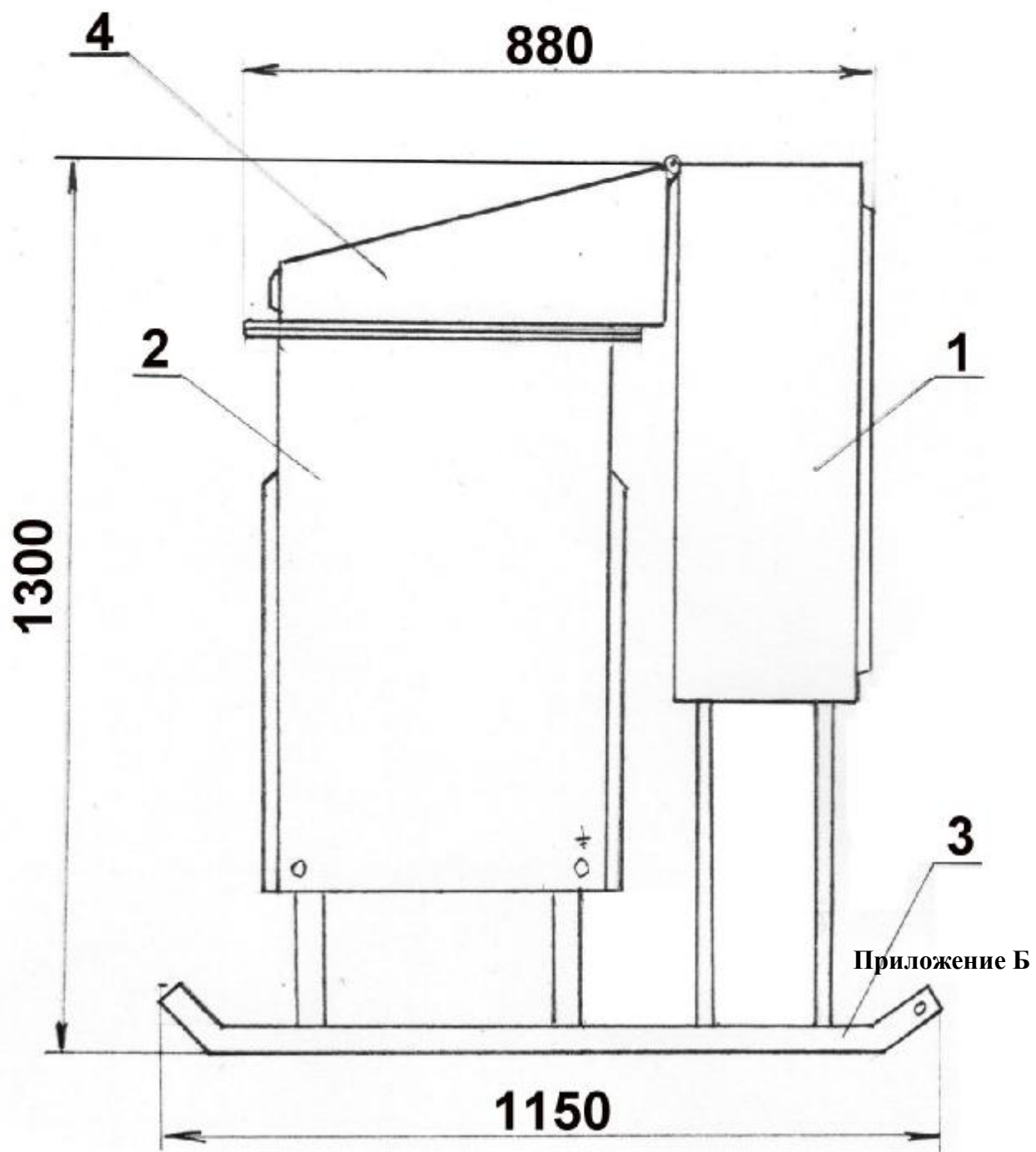
Рис.1 Комплексная трансформатная подстанция КТПТО-80-У1
